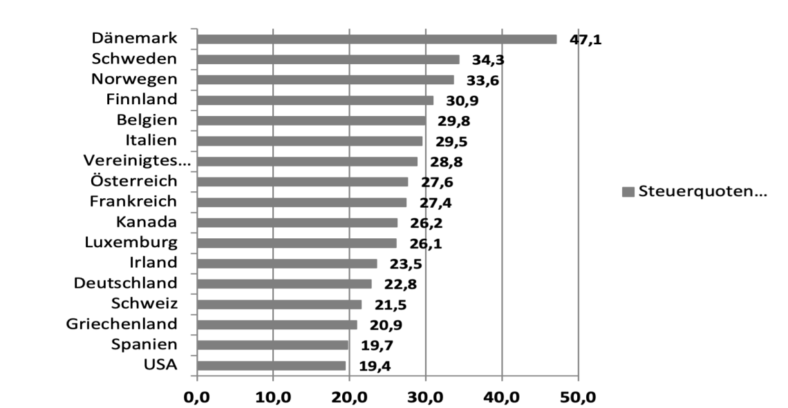
Abbildung 1: Steuerquoten im internationalen Vergleich
